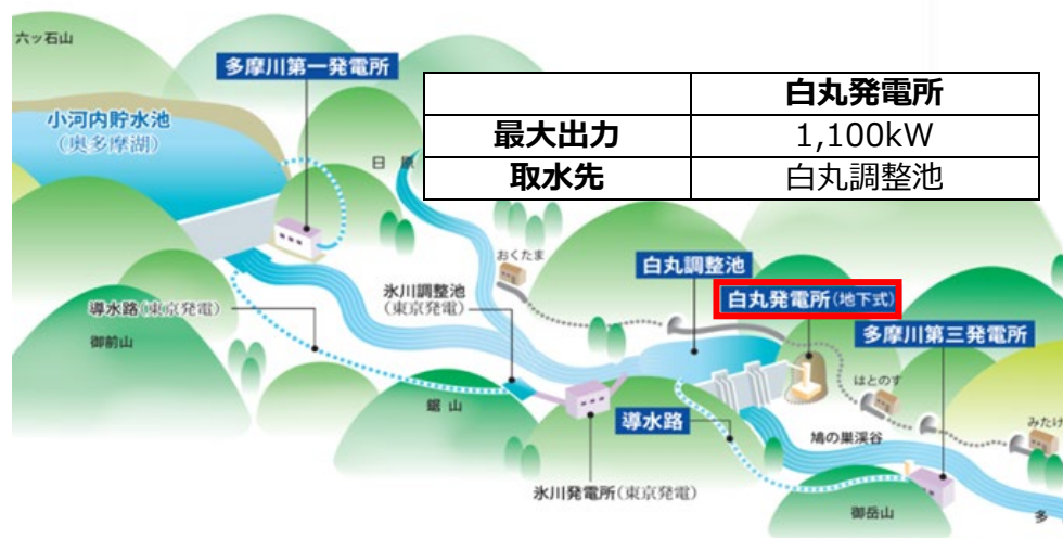
多摩川水系の水力発電事業概要
