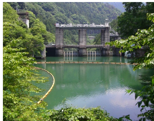
白丸調整池ダム
