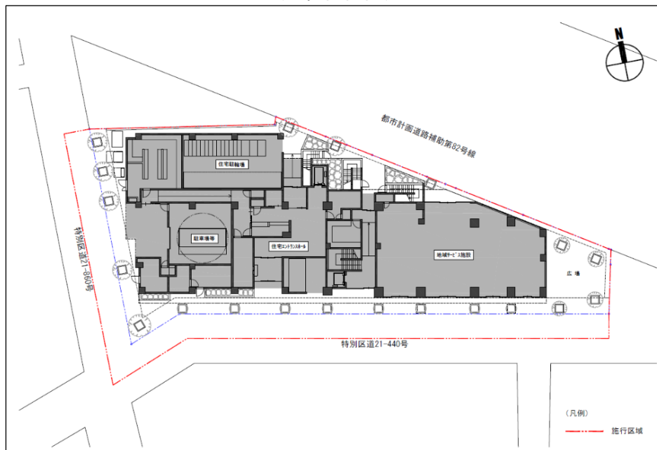
(配置計画図)
