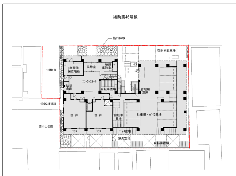
(配置計画図)
