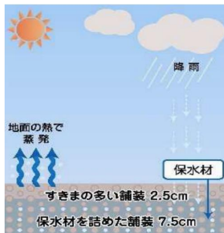
【保水性舗装の仕組み】
