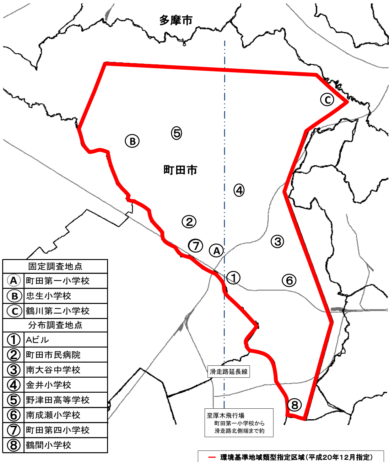
図3 平成30年度厚木飛行場騒音調査地点図
