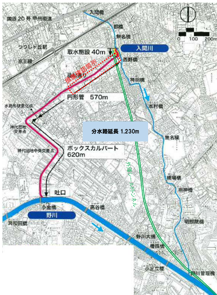
入間川分水路平面図
