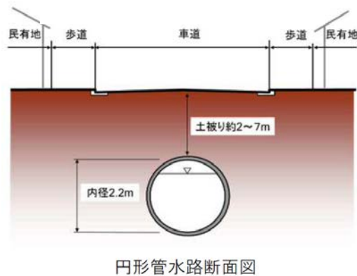
入間川分水路断面図
