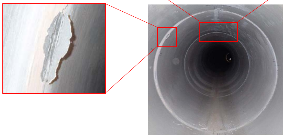
管渠目地モルタル剥離等の一例 (写真)
