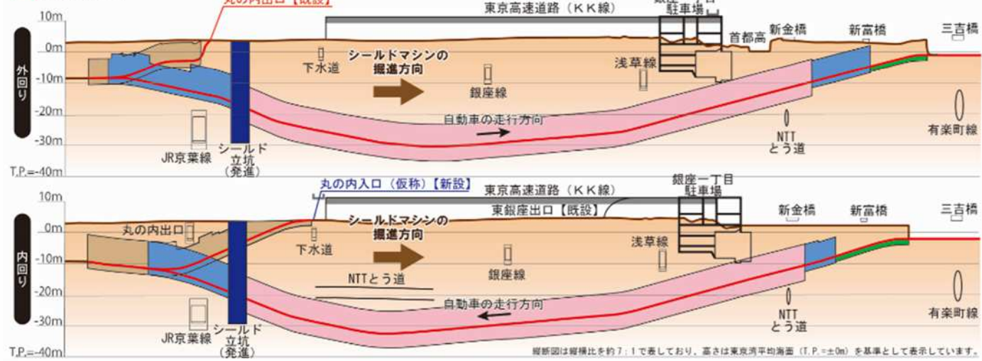
縦断模式図
