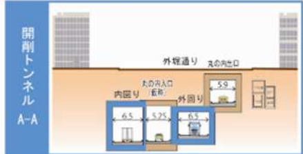
横断模式図
